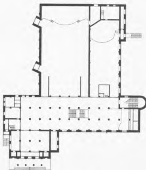
▲ План 1 этажа
