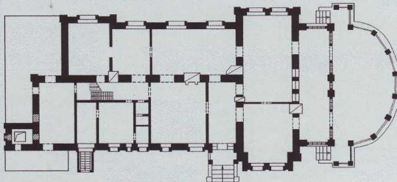
▲ План 1 этажа дома Рутгерса (обмеры: Н. С. Филина, 1993)
